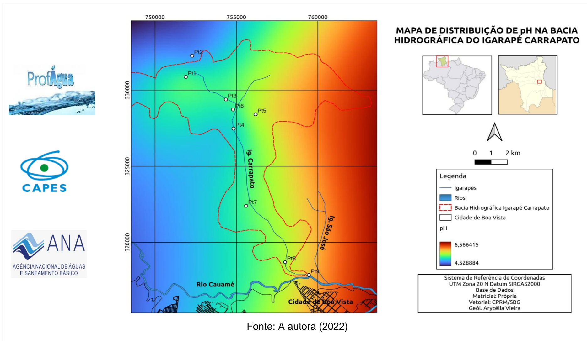
Figura 19 – Mapa de distribuição do pH na BHIC.
