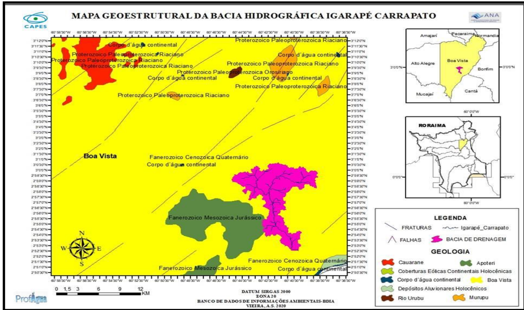
Figura 4– Mapa Geológico e geoestrutural da área da bacia hidrográfica do Igarapé Carrapato, evidenciando a estruturação da área da bacia sedimentar do Tacutu.
