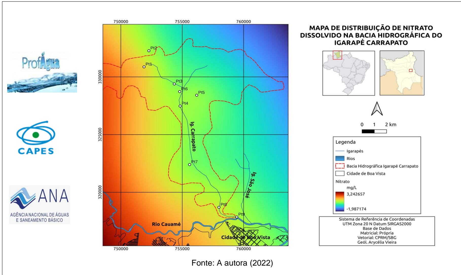
Figura 17 – Mapa de Distribuição do Nitrato.
