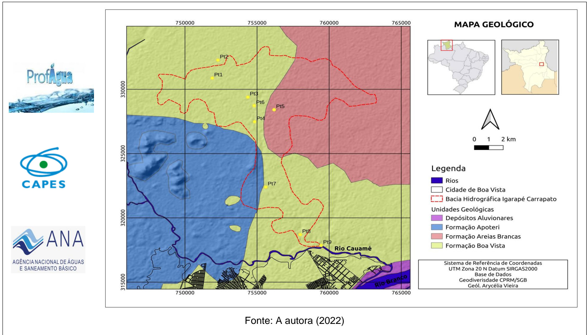
Figura 35 – Mapa geológico da área da BHIC.
