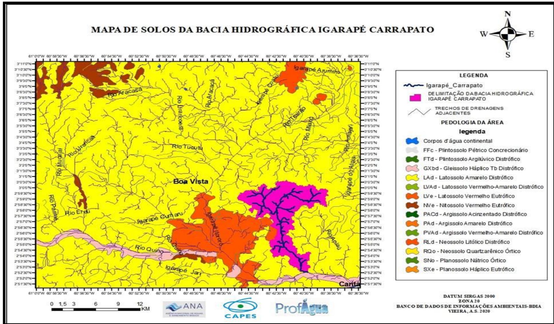
Figura 5– Mapa de solos da Bacia Hidrográfica Igarapé Carrapato.
