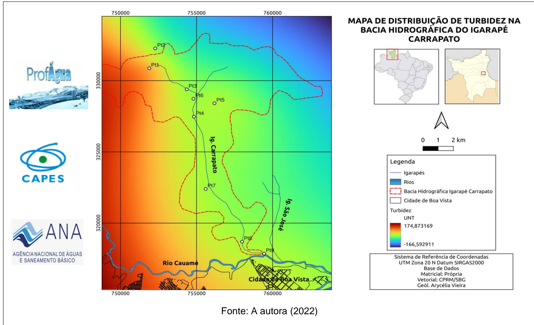
Figura 22 – Mapa de distribuição da Turbidez na BHIC.
