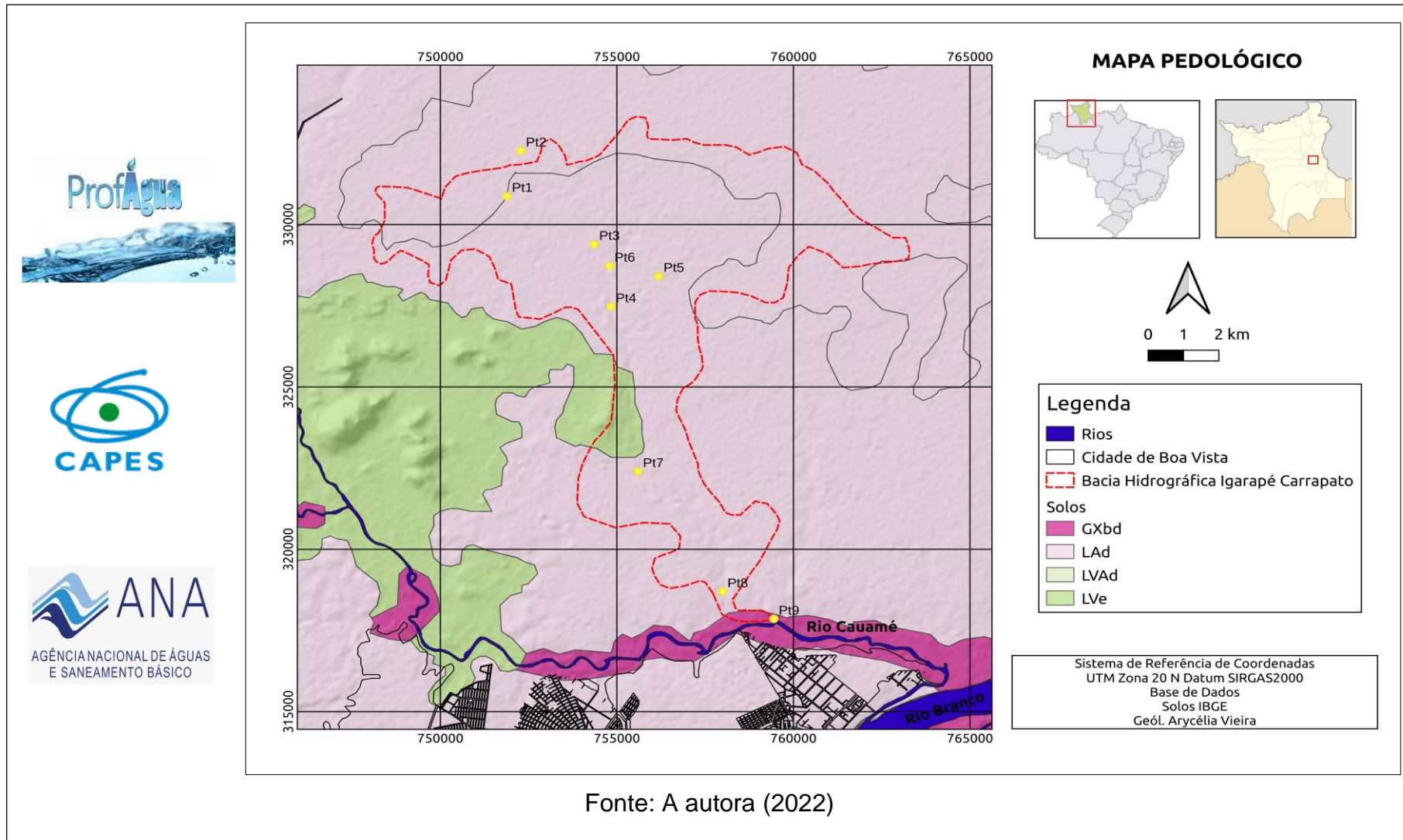
Figura 11– Mapa Pedológico da área da BHIC.
