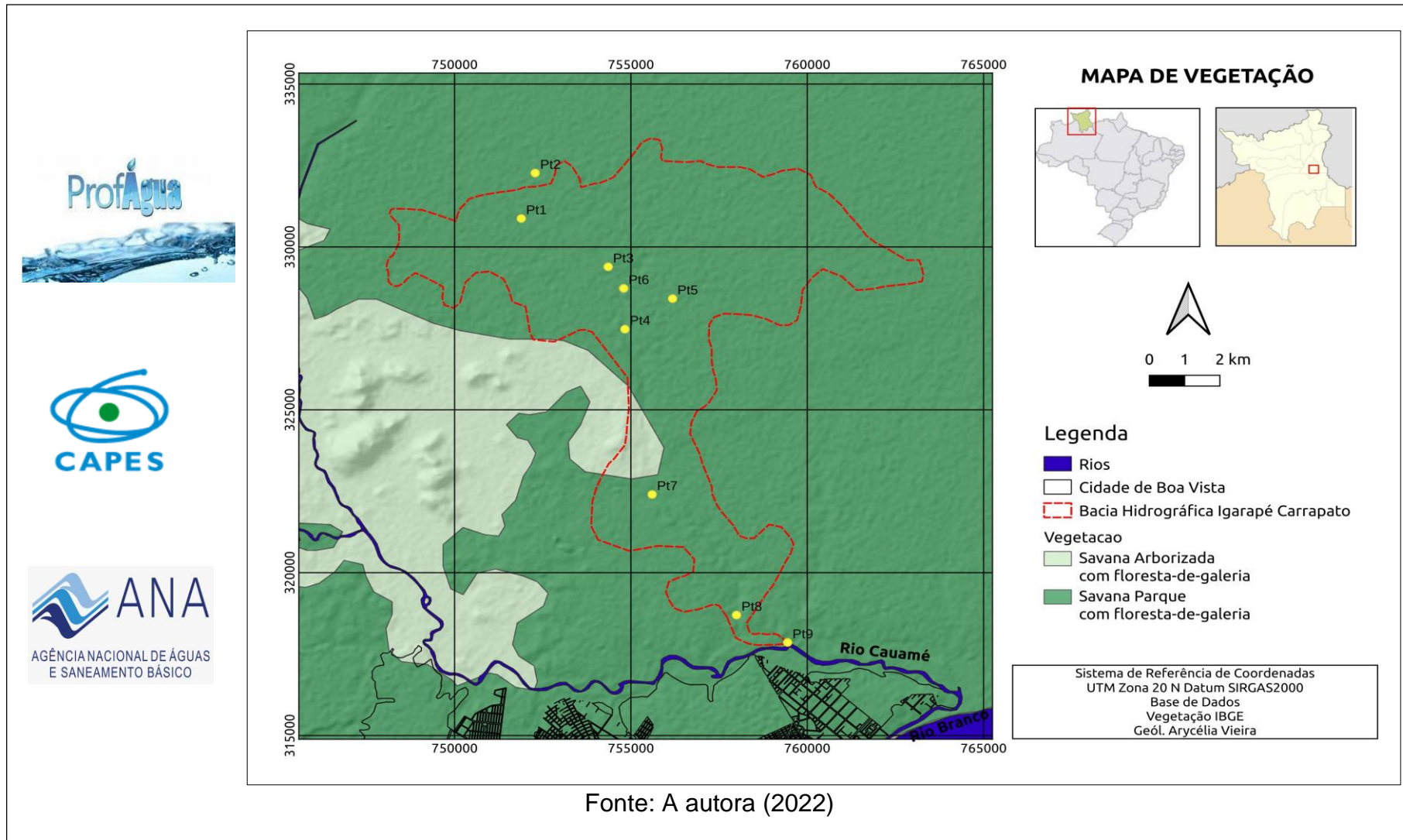
Figura 12 – Mapa de Vegetação da BHIC.
