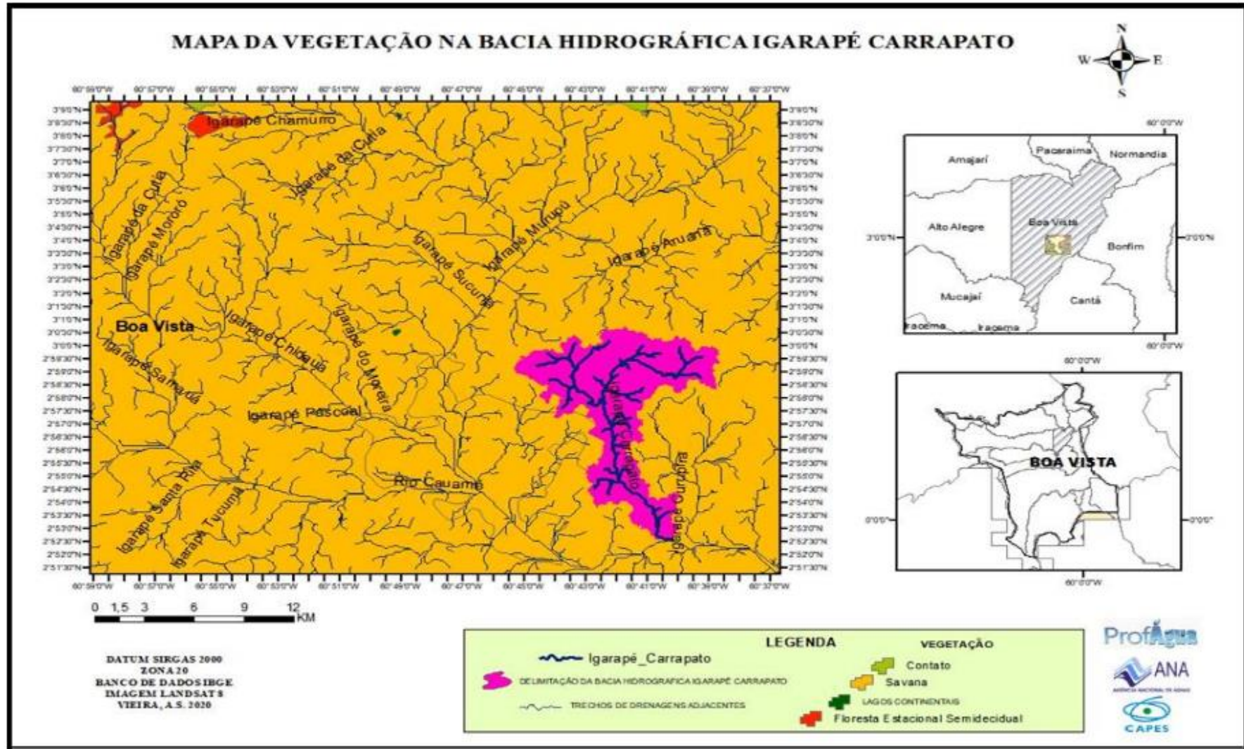
Figura 7 – Mapa de vegetação da bacia hidrográfica Igarapé Carrapato, mostrando toda sua área de influência inserida dentro de uma área de Savana.
