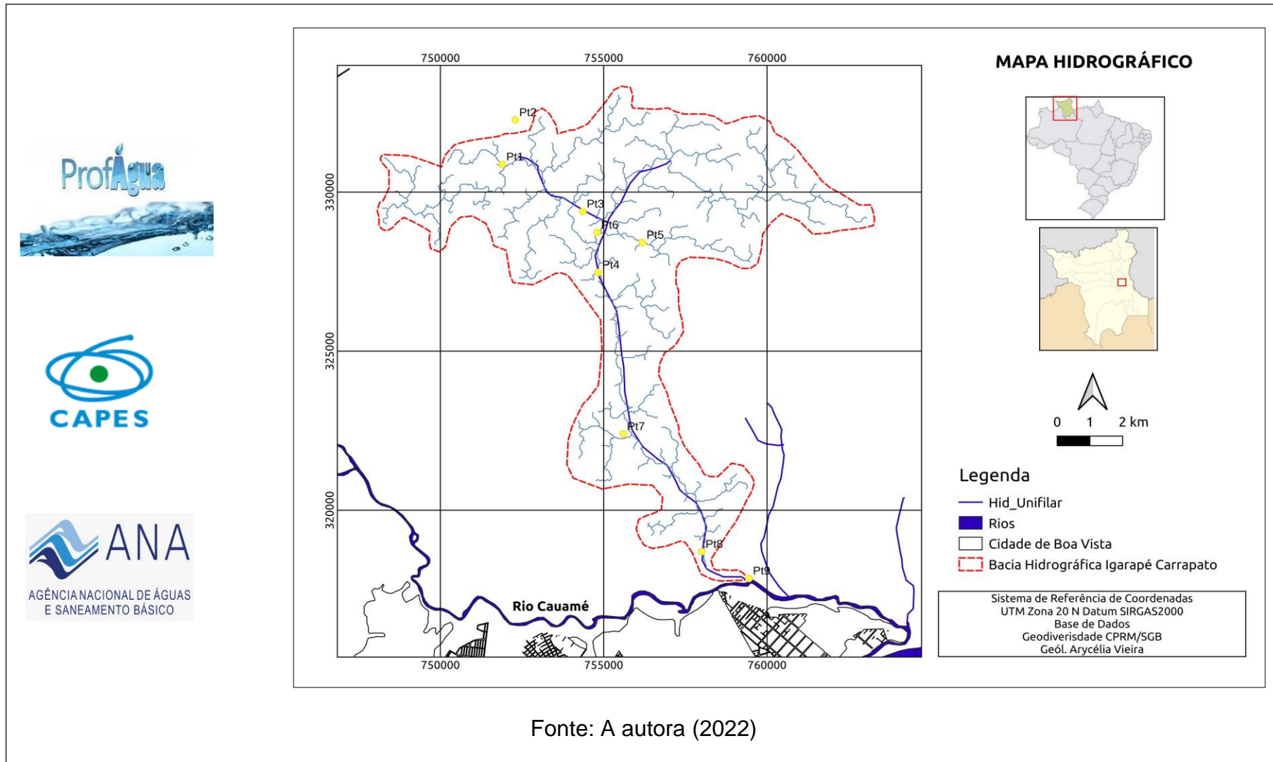
Figura 13 – Mapa hidrográfico da BHIC.
