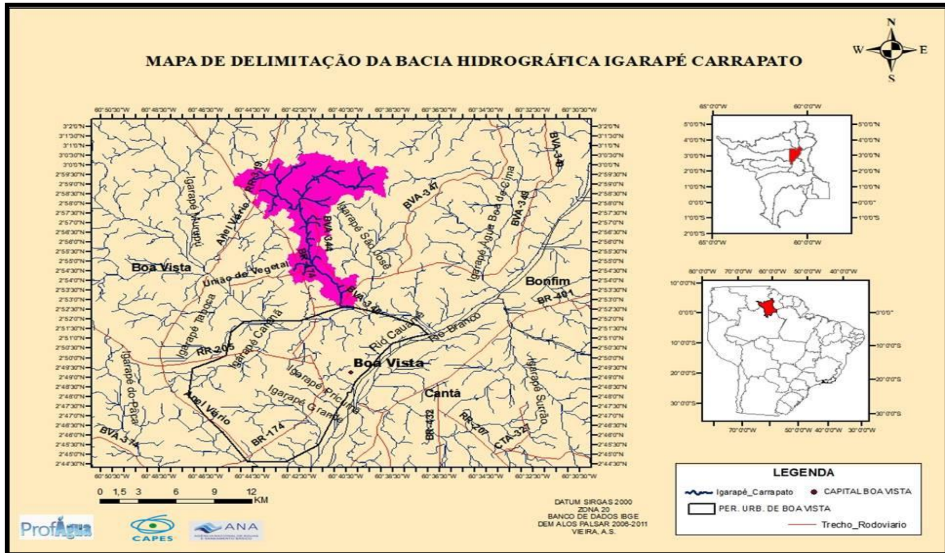
Figura 6– Mapa hidrográfico da região de estudo e delimitação da Bacia Hidrográfica Igarapé Carrapato.
