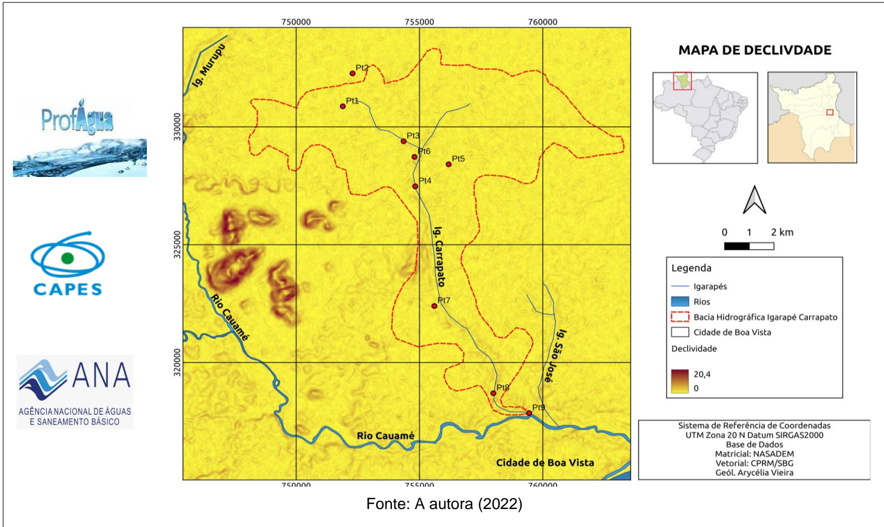
Figura 9 – Mapa de declividade da BHIC.
