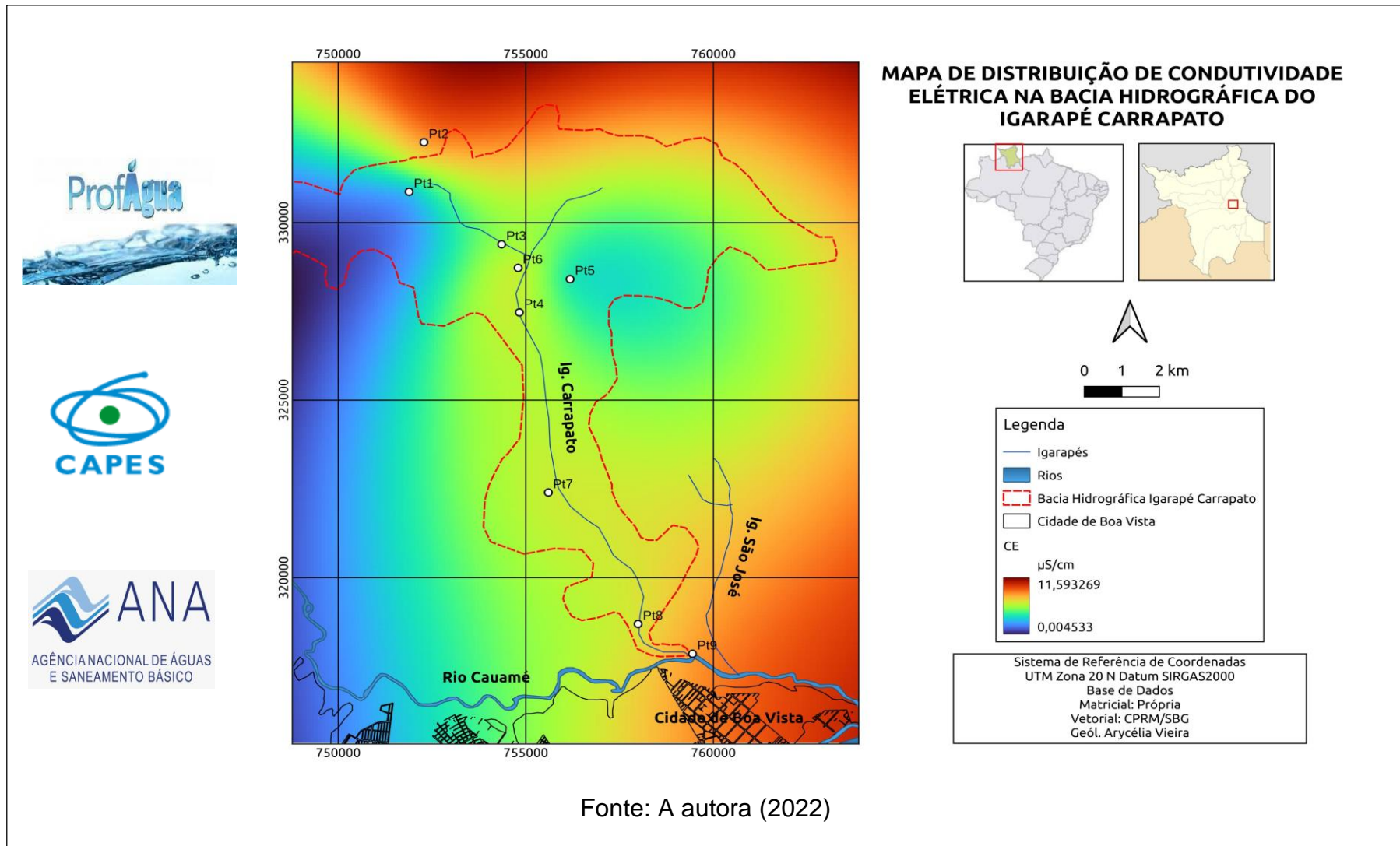
Figura 23 – Mapa de distribuição da Condutividade Elétrica na BHIC.
