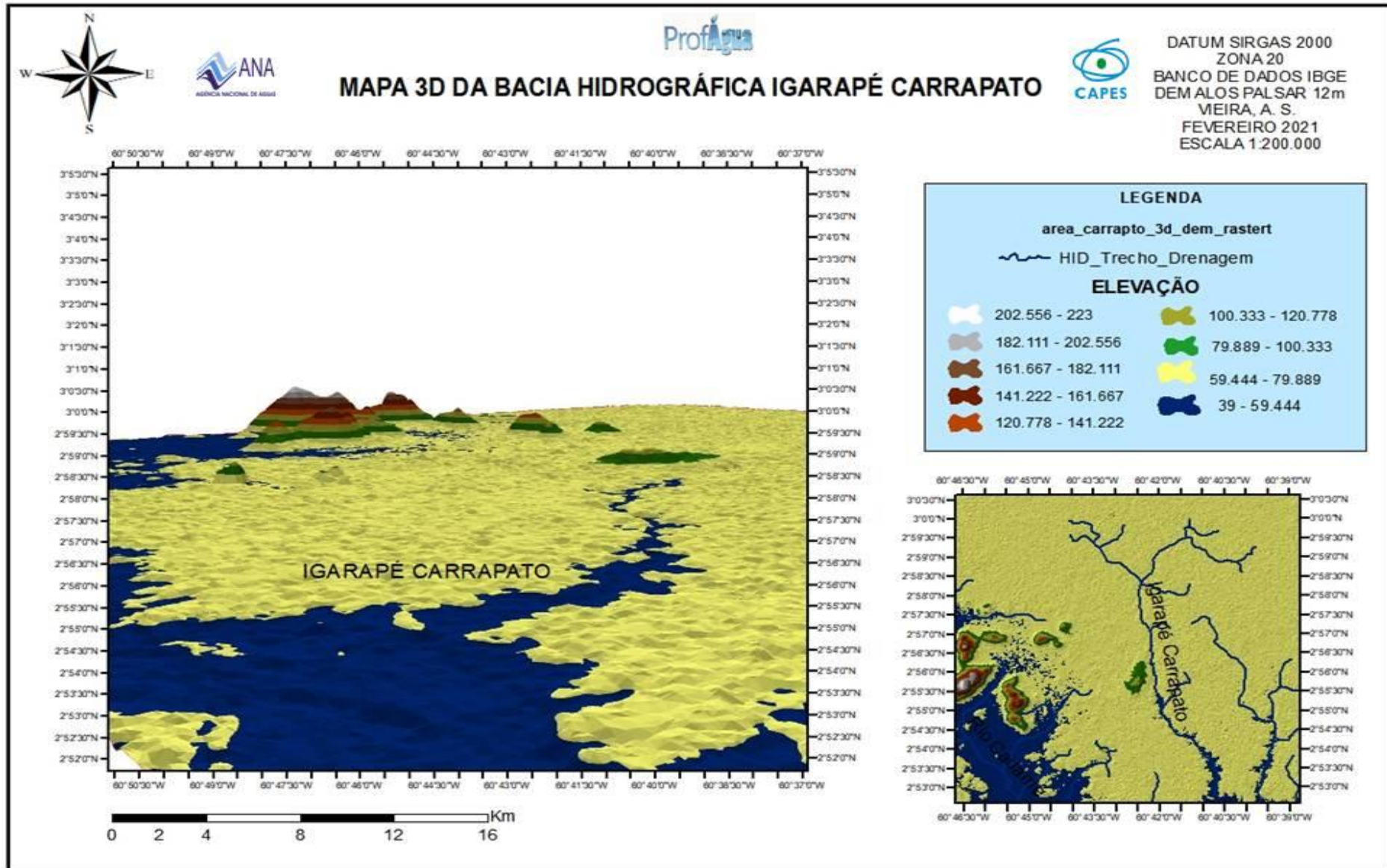
Figura 3– Mapa 3D da bacia e modelagem dimensional da elevação altimétrica.
