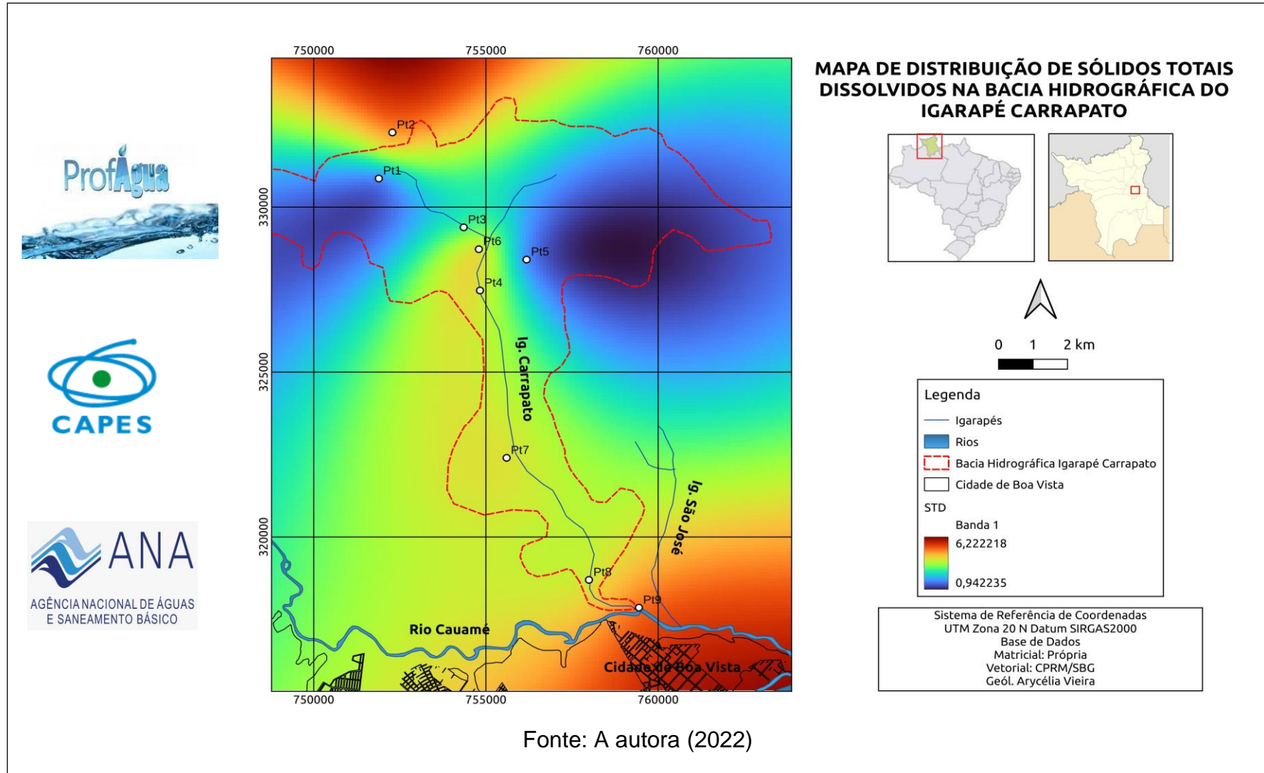
Figura 21– Mapa de distribuição dos Sólidos Totais Dissolvidos na BHIC.
