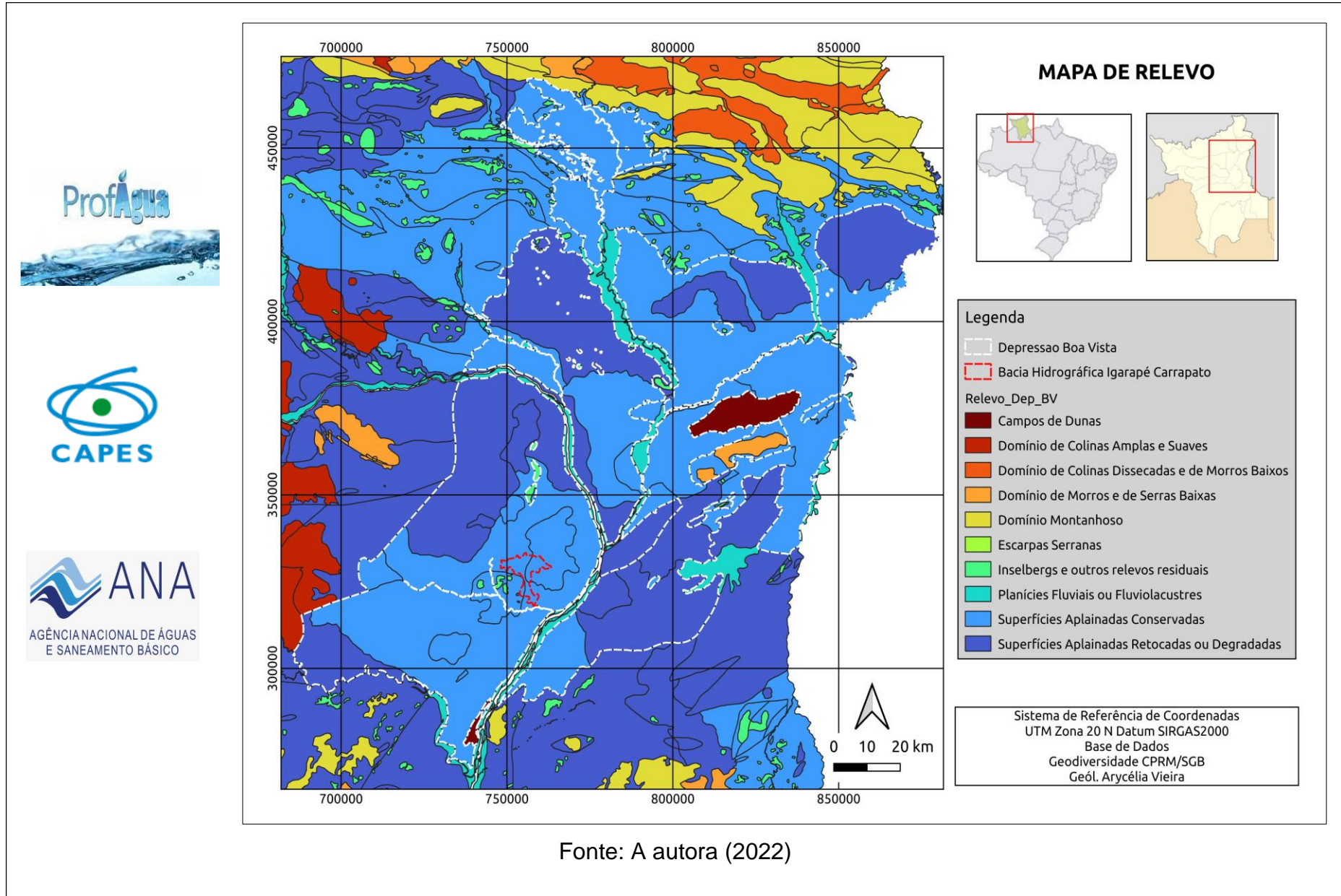
Figura 1 – Mapa da Depressão Boa Vista e relevo associado.
