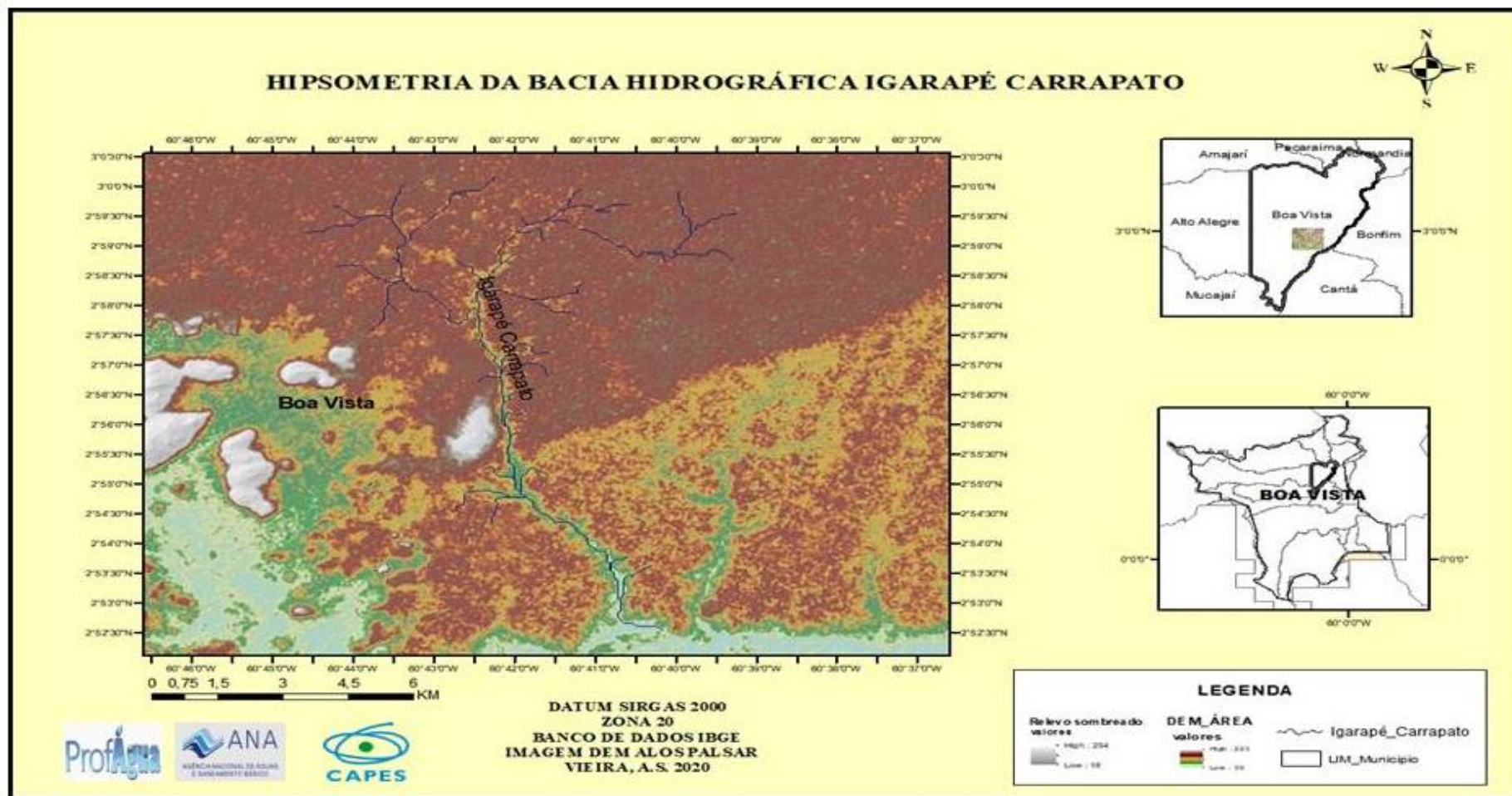
Figura 2– Mapa Hipsométrico da bacia hidrográfica Igarapé Carrapato, evidenciando essas áreas planas.
