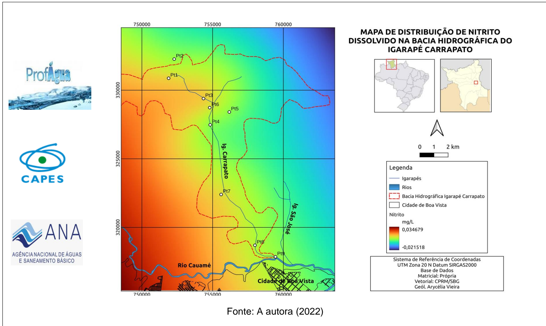
Figura 16– Mapa de distribuição do Nitrito.
