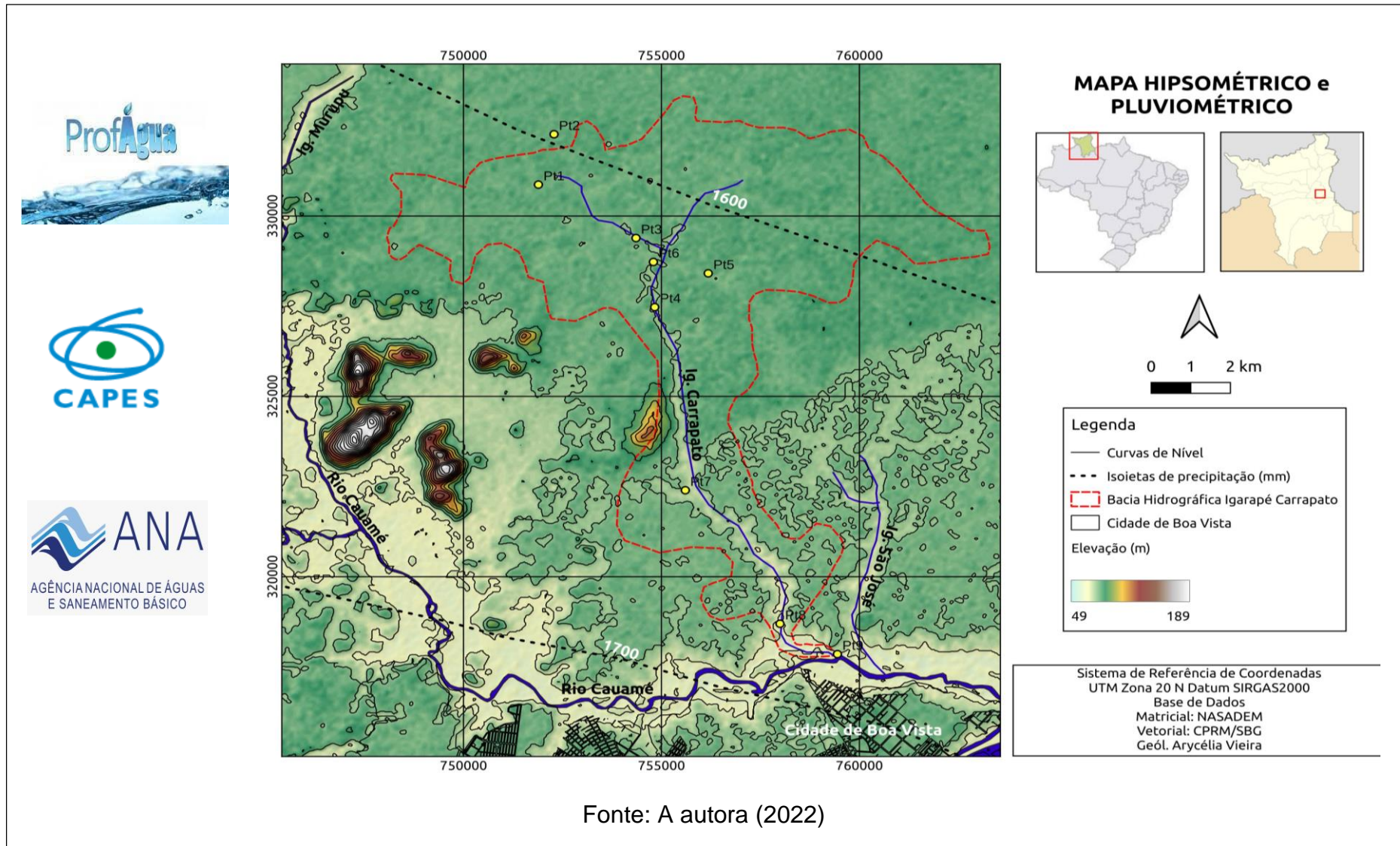
Figura 8 – Mapa Hipsométrico e Pluviométrico da BHIC.
