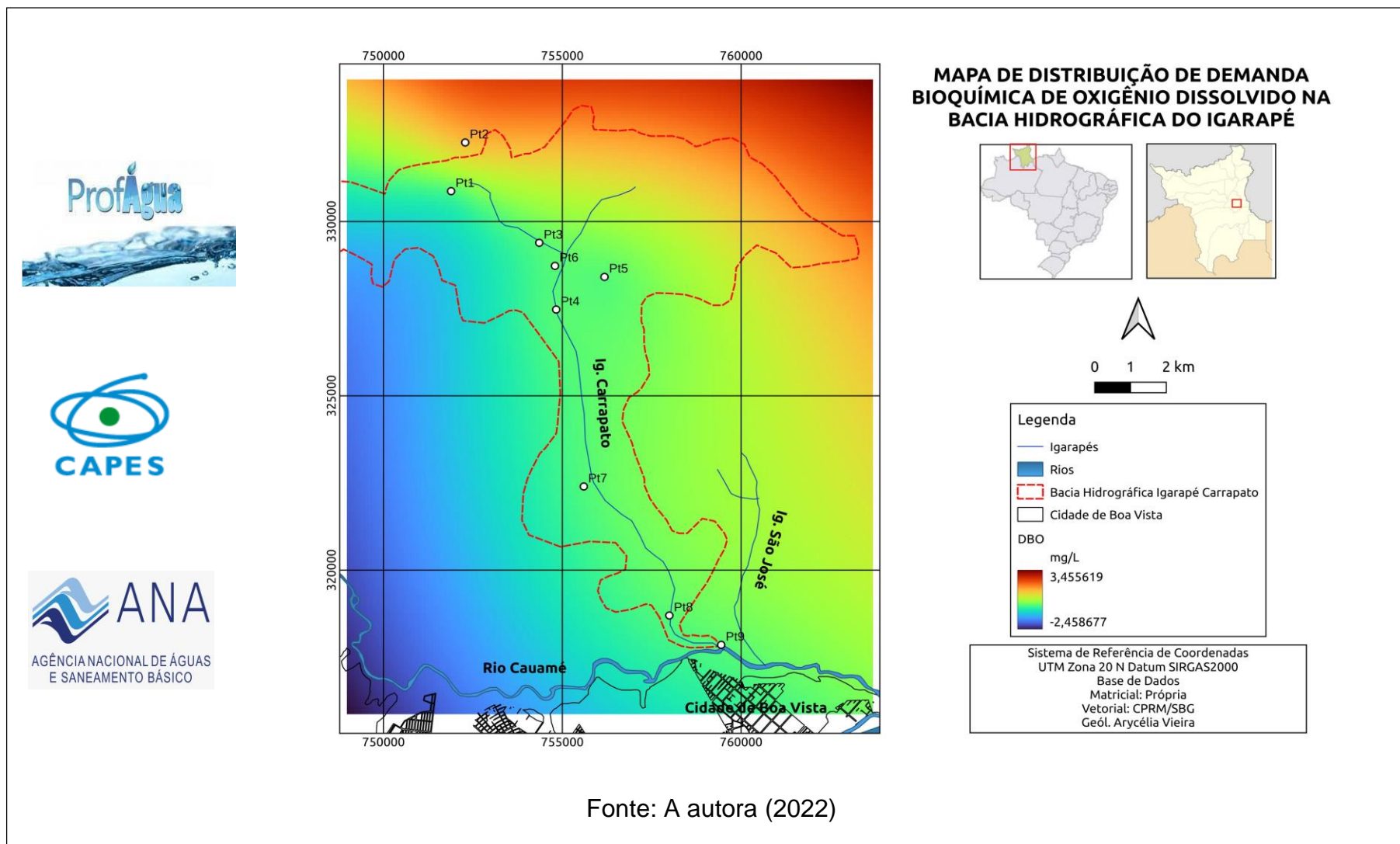
Figura 18 – Mapa da distribuição de DBO 5,20 na BHIC.
