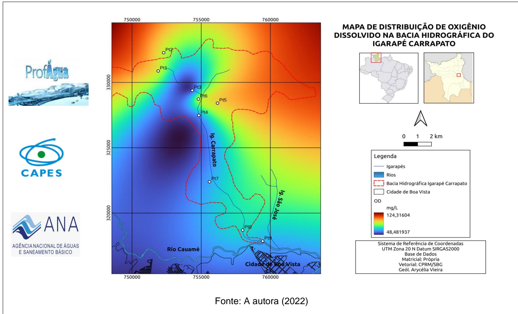
Figura 20– Mapa de distribuição do Oxigênio Dissolvido na BHIC.
