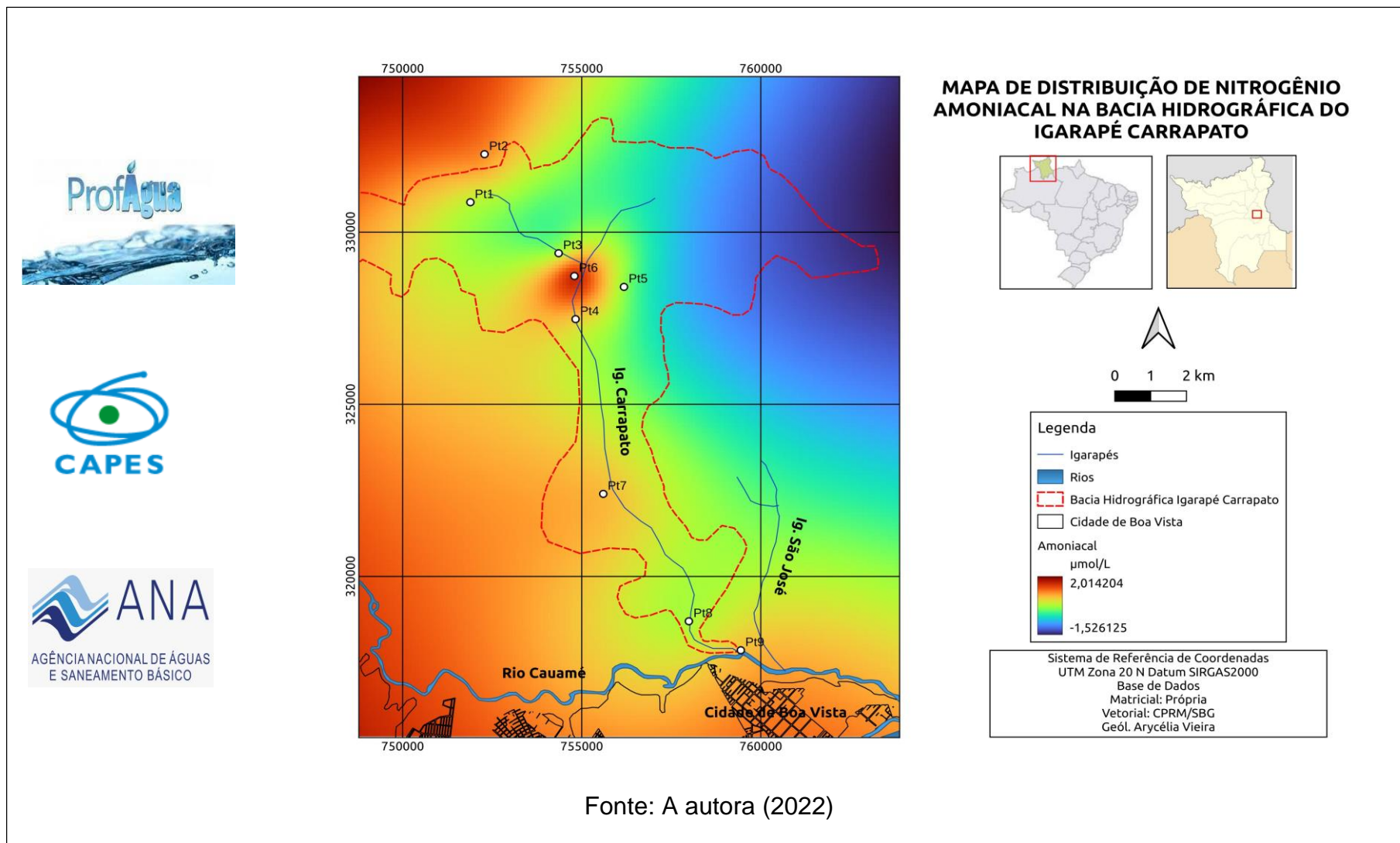
Figura 15Figura 41 – Mapa de distribuição do Nitrogênio Amoniacal na BHC.
