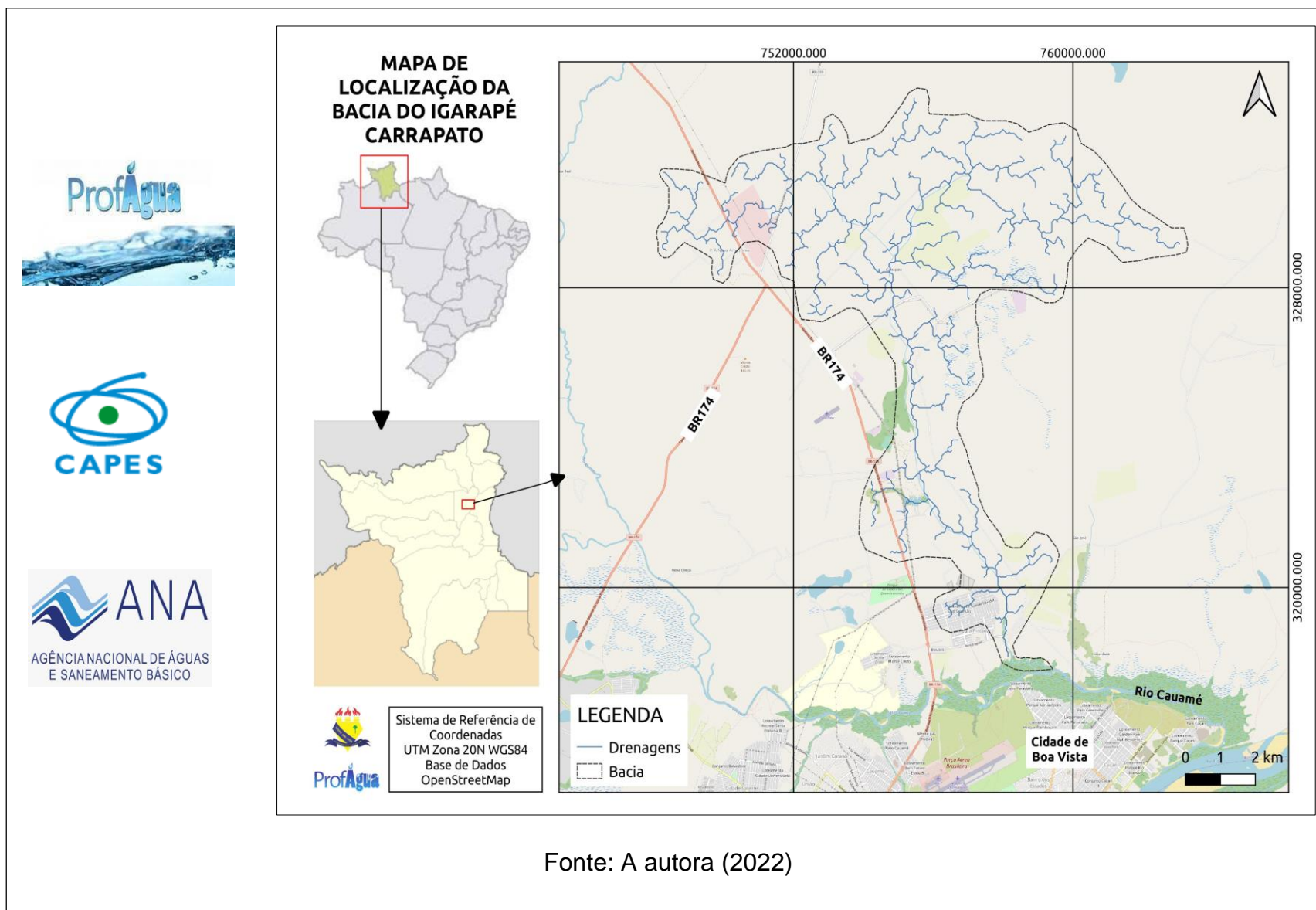
Figura 09- Mapa de localização da bacia hidrográfica Igarapé Carrapato, Boa Vista, Roraima. Fonte: Autora (2022).
