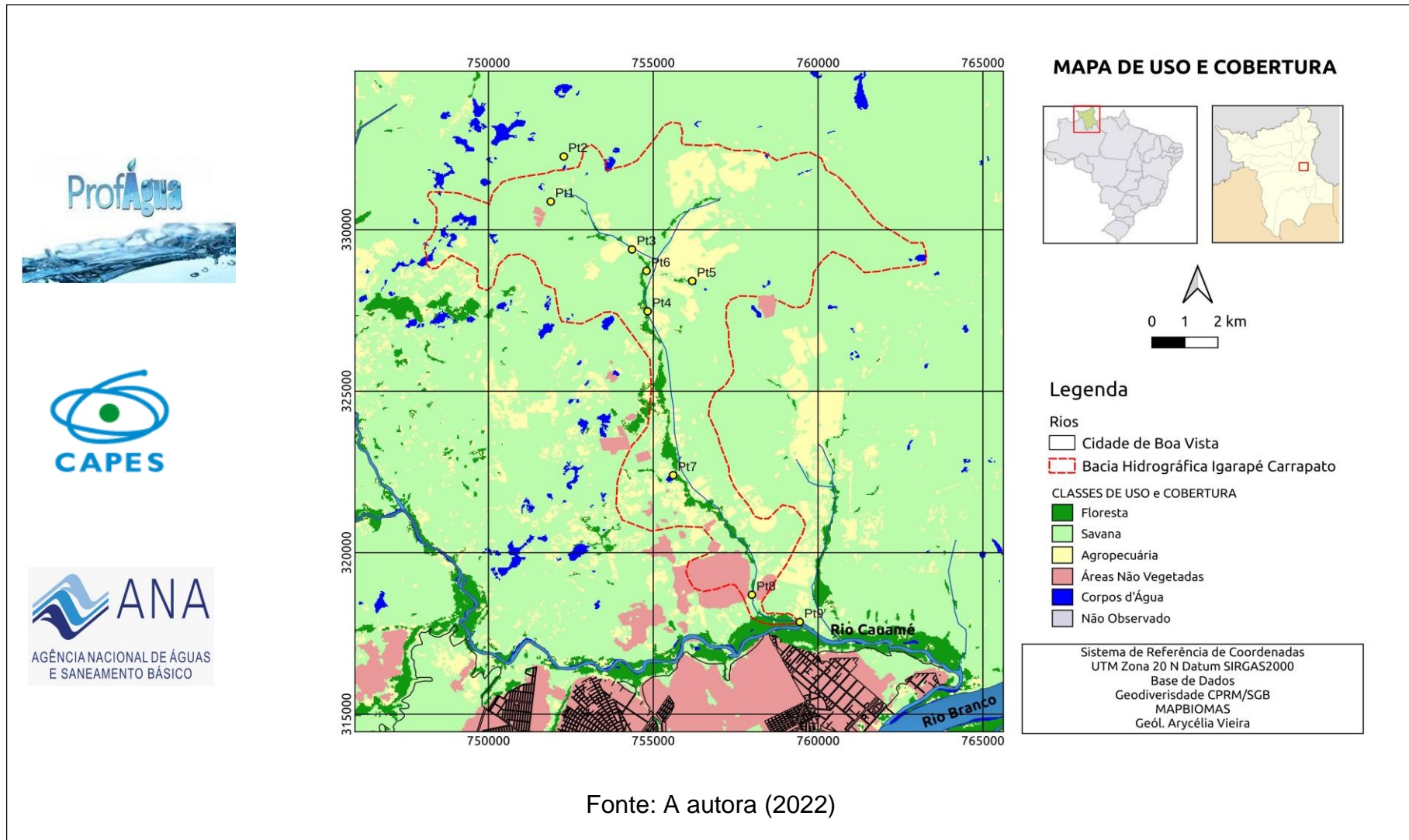
Figura 14 – Mapa de uso e cobertura do solo da BHIC.
