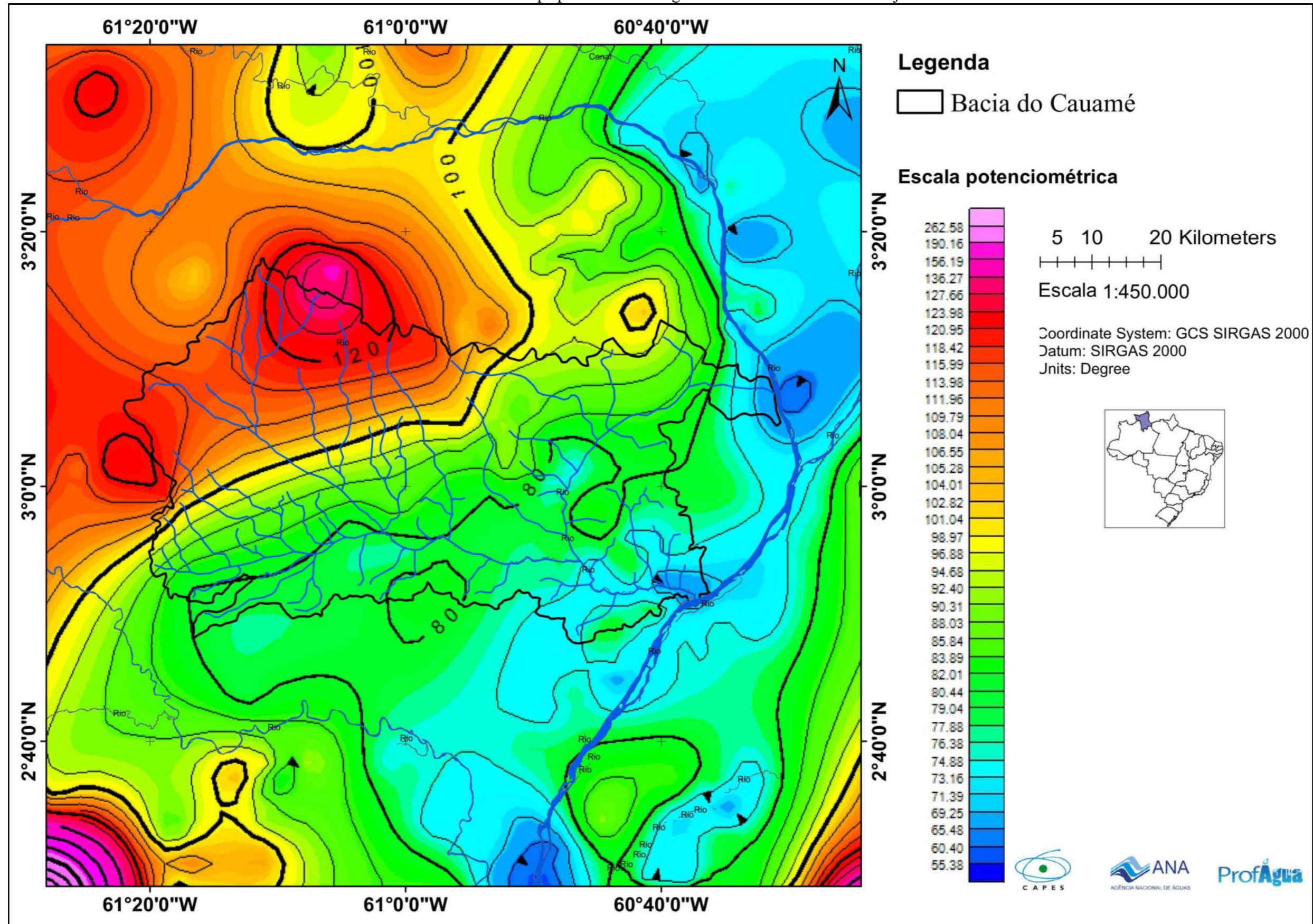
ANEXO G – Mapa potenciométrico gerado no Software Oasis Montaj
