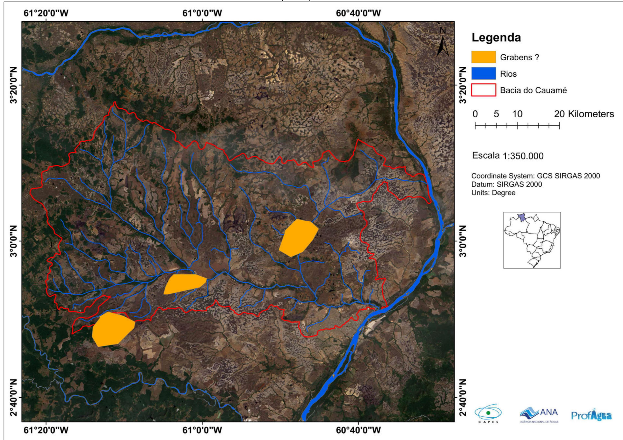
ANEXO K - Mapa com possíveis Horsts e Grabens
