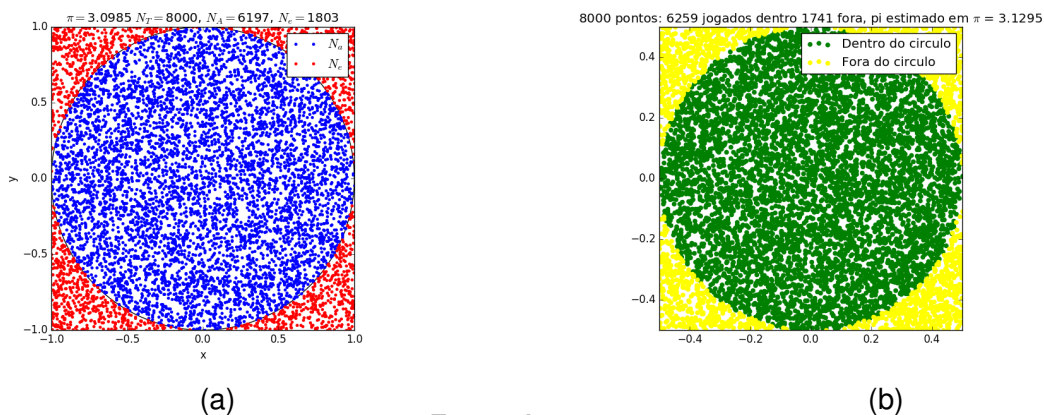
Figura 26: 8000 dardos lançados no alvo.
