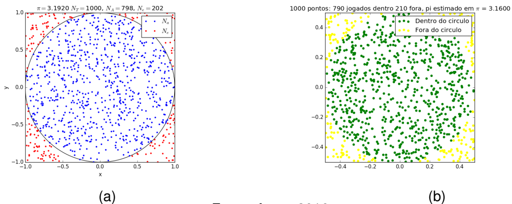
Figura 25: 1000 dardos lançado no alvo.
