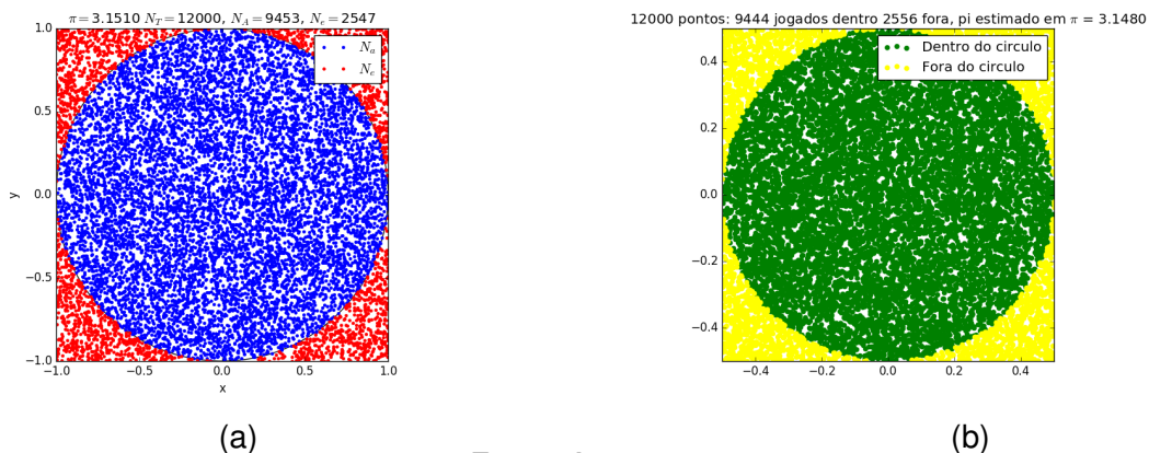
Figura 27: 12000 dardos lançados no alvo.
