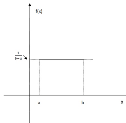
Figura 14: Função distribuição de probabilidade uniforme para variável aleatória contínua
